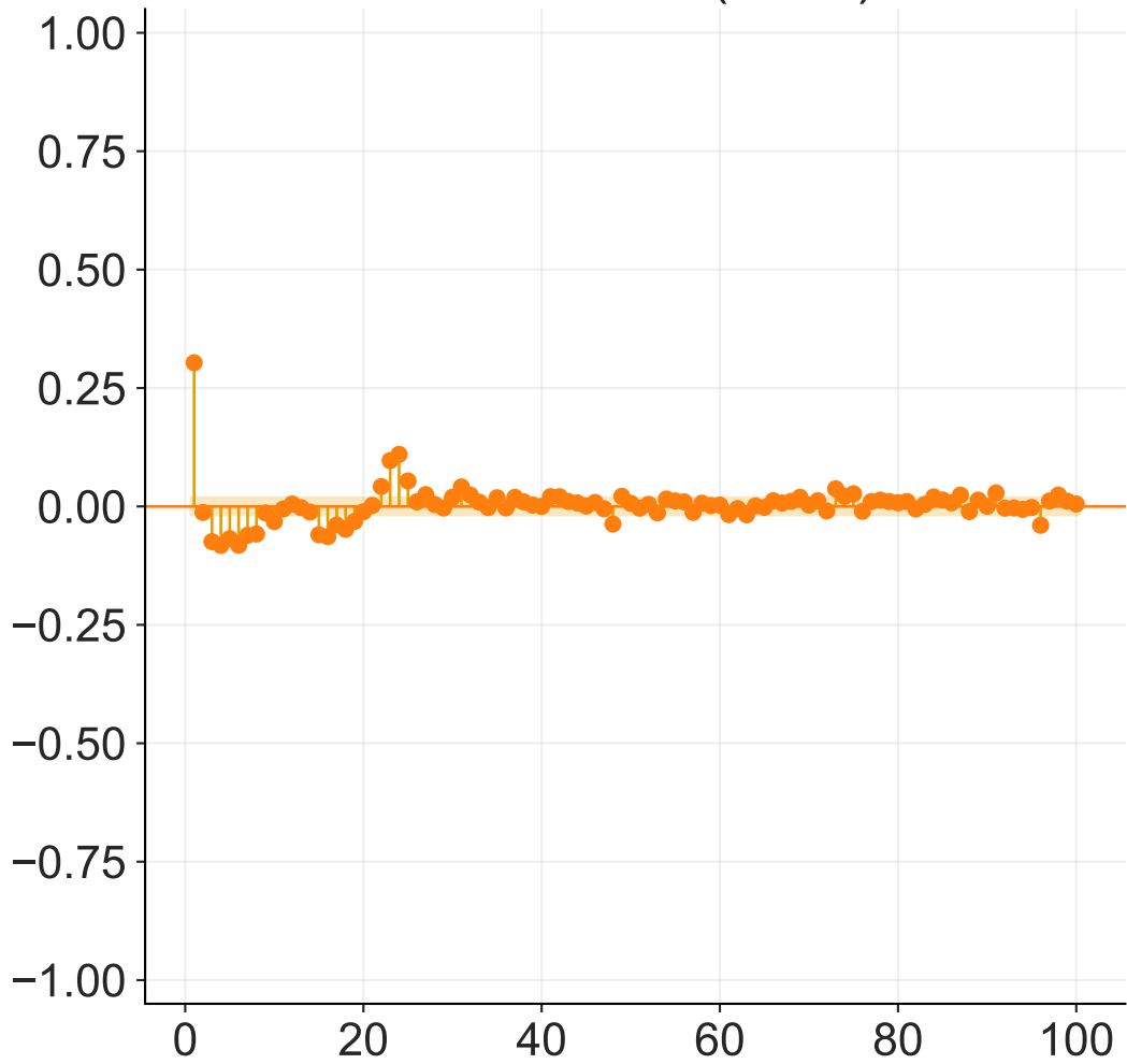
PACF MSM (2020)
